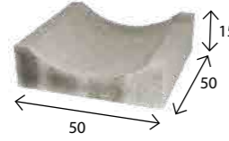
Korytko ściekowe 50/50/15
