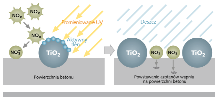
Mechanizm oczyszczania powietrza z tlenków azotu NO x przez aktywną fotokatalityczną powierzchnię kostki brukowej wykonaną z użyciem cementu TioCem®
