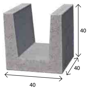
Korytko górskie 40/40/40
