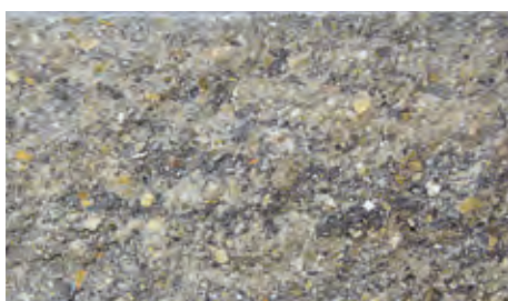
Andezit
