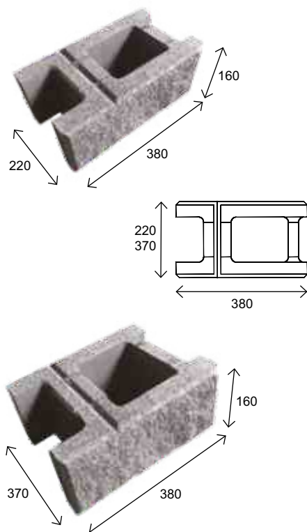
Blok múrikový 370
