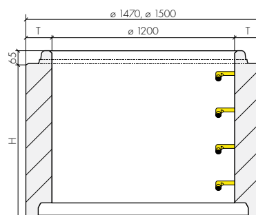
Šachtová skruž so zámkom (Q)
