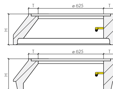
Šachtová skruž - kónus so zámkom (Z)
