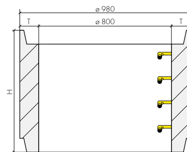
Šachtová skruž so zámkom (Z)
